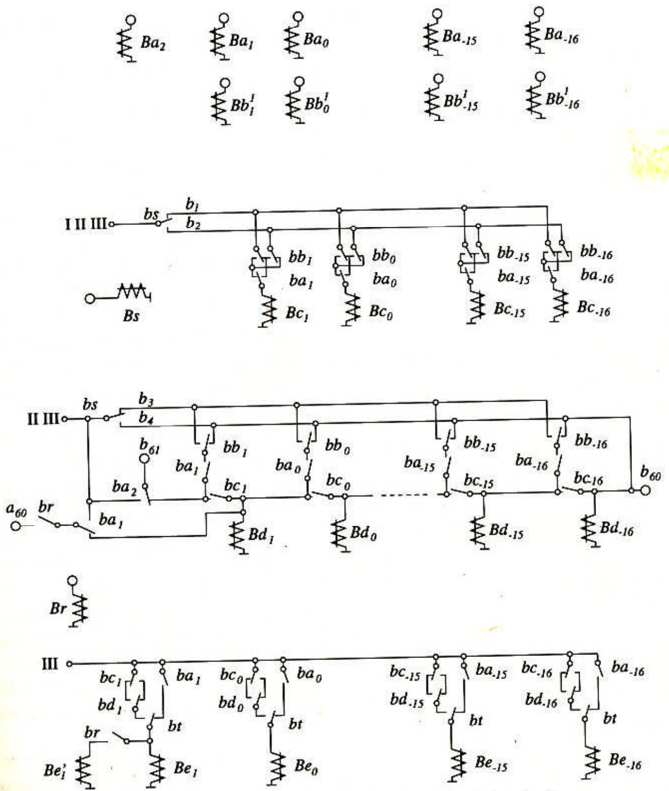
Abbildung 4. Additionswerk (Teil B für Mantisse)
